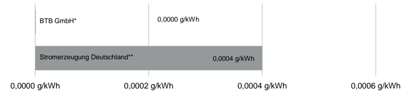
Radioaktiver Abfall
