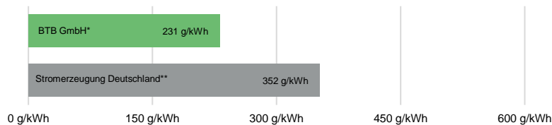
CO 2 -Emissionen
